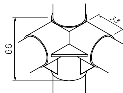
JUNTA DE PLÁSTICO TIPO 3 VIAS
