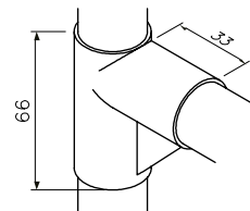
JUNTA DE PLÁSTICO TIPO 2 VIAS
