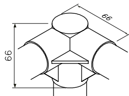
JUNTA DE PLÁSTICO SUPERIOR TIPO PLANA
