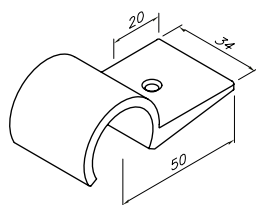
GRAMPO DE TUBO DE JUNTA DE PLÁSTICO
